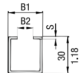
Tragschiene TS-30
